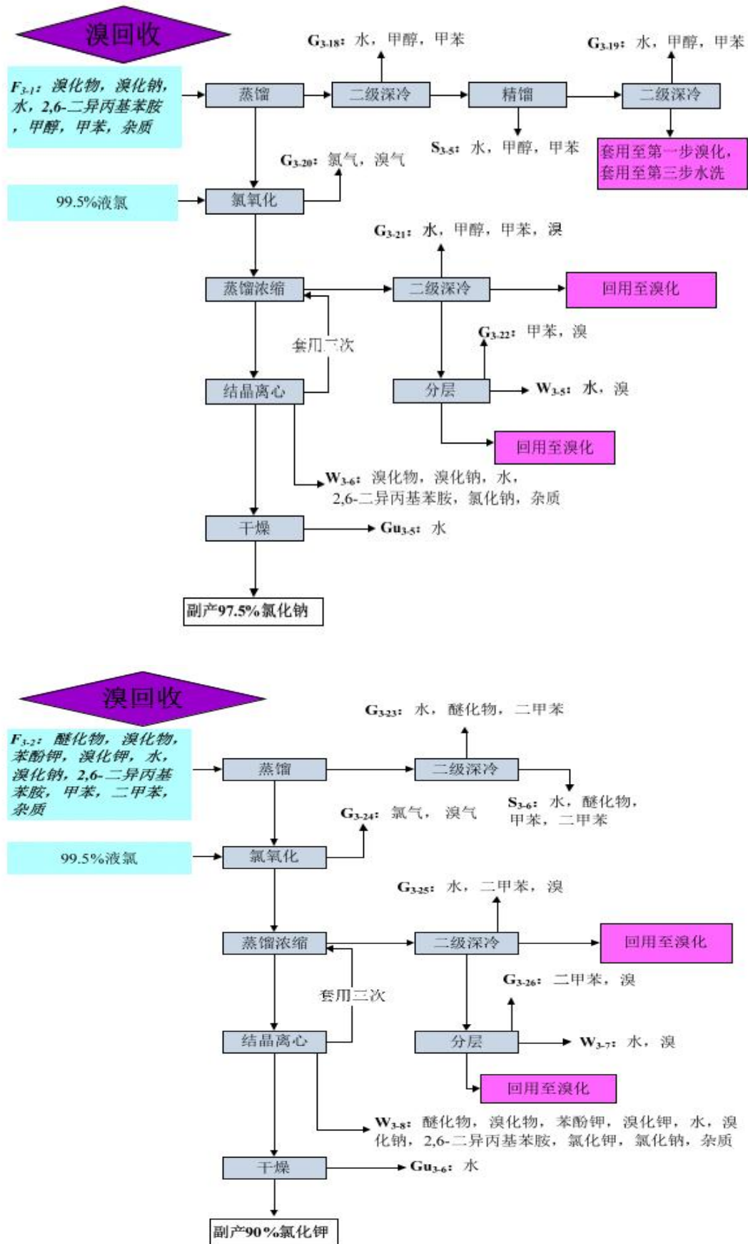
图 4.3-7 丁醚脲生产工艺流程图
